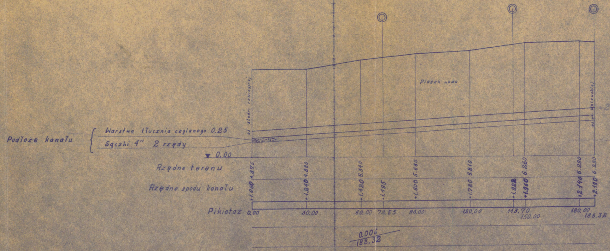
Profil podłużny kan. z rur kam. \phi 0.40 na ul. Świętosławskiej odc. od ul. Suchodolskiej do ul. Walewskiej 1: 1000 pozioma 100 pionowa
